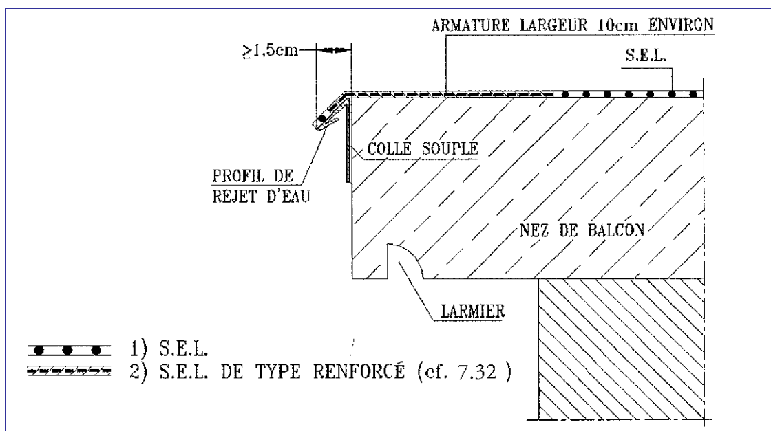
Figure 4 : Exemple d'exécution en rive plate avec débord
